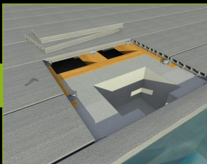
Trappe invisible rendue accessible par le cavalier et sa came 45°
