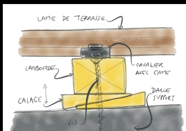
Pose sur dalle + lambourdes
