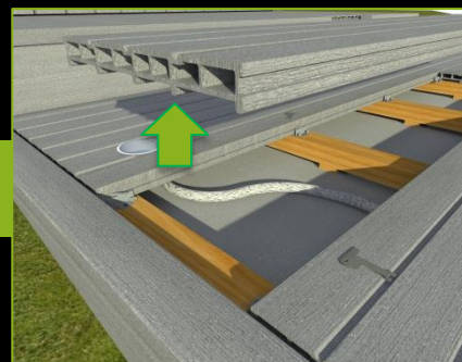
Vide technique visitable pour entretien de l'étanchéité par démontage unitaire des lames
