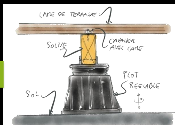
Pose sur sol + plots
