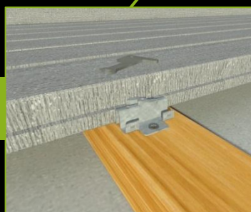
Pose sur lambourdes
